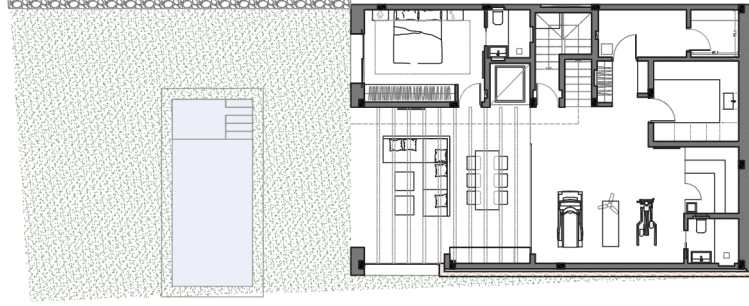
PLANTA SOTANO
