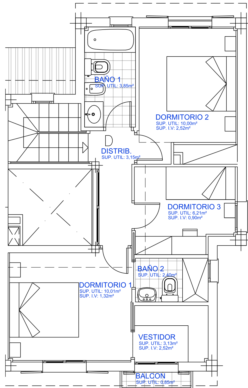
PLANTA ALTA
