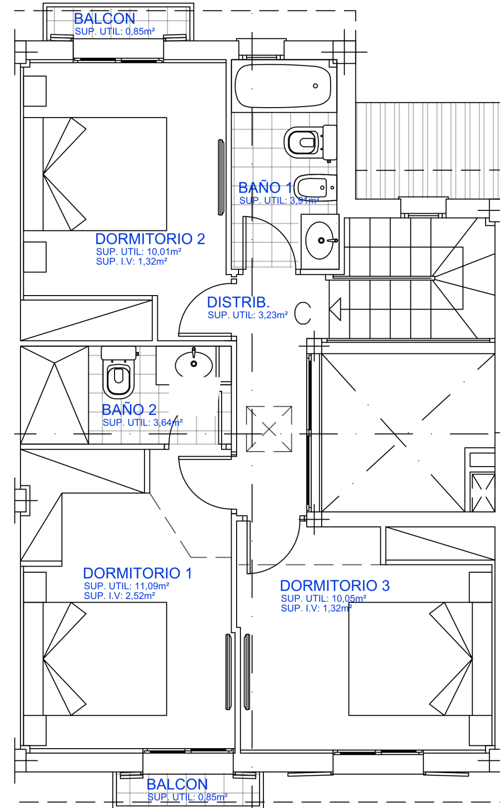
PLANTA ALTA
