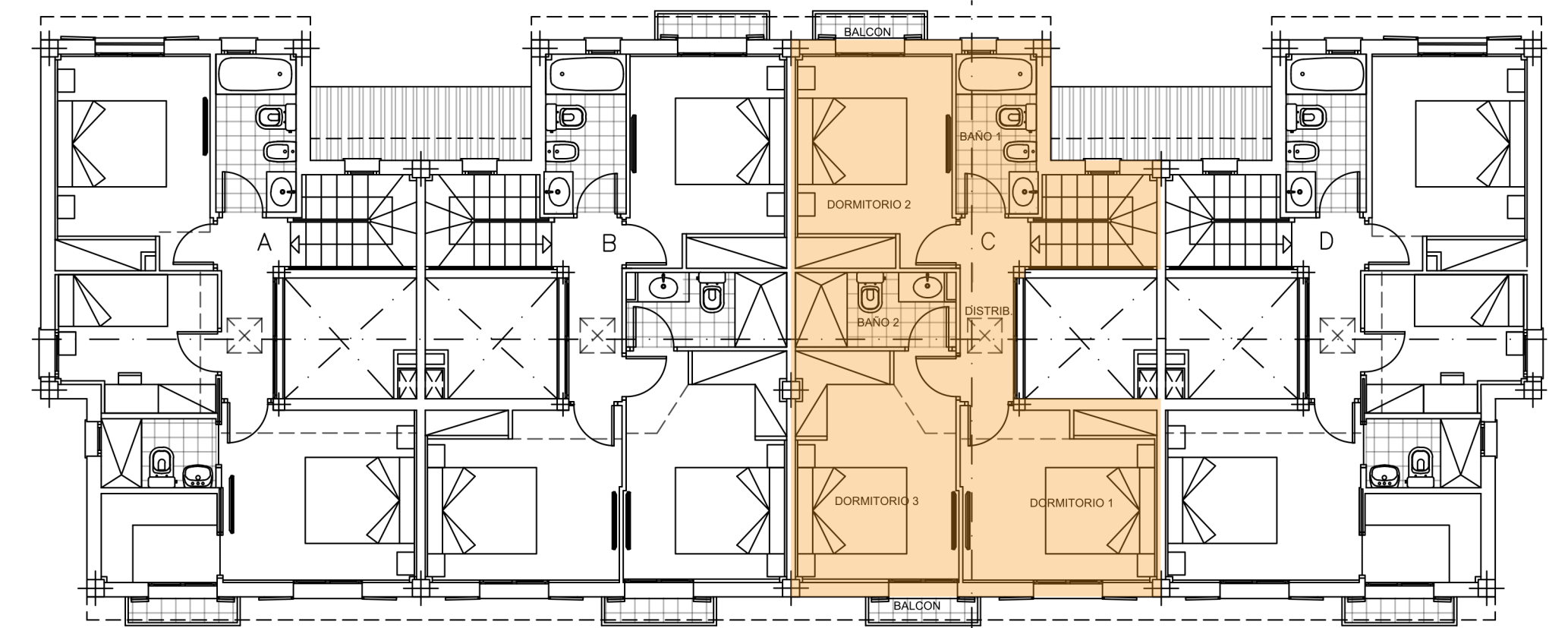
PLANTA ALTA
