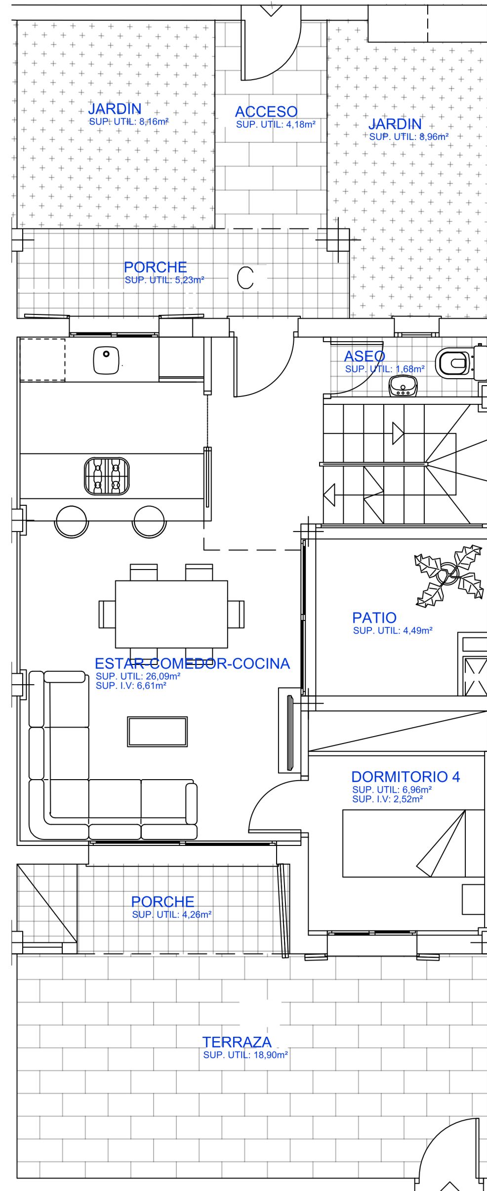
PLANTA BAJA
