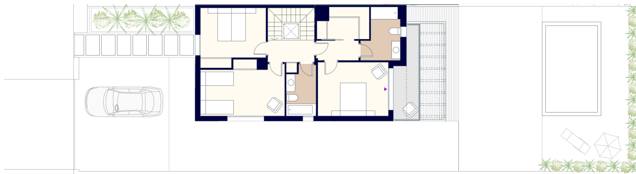
Planta primera
